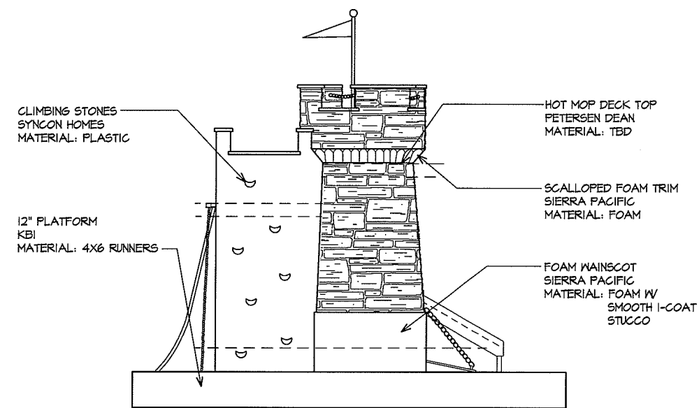
LEFT ELEV.
