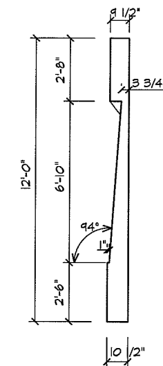
SECTION 'A'
